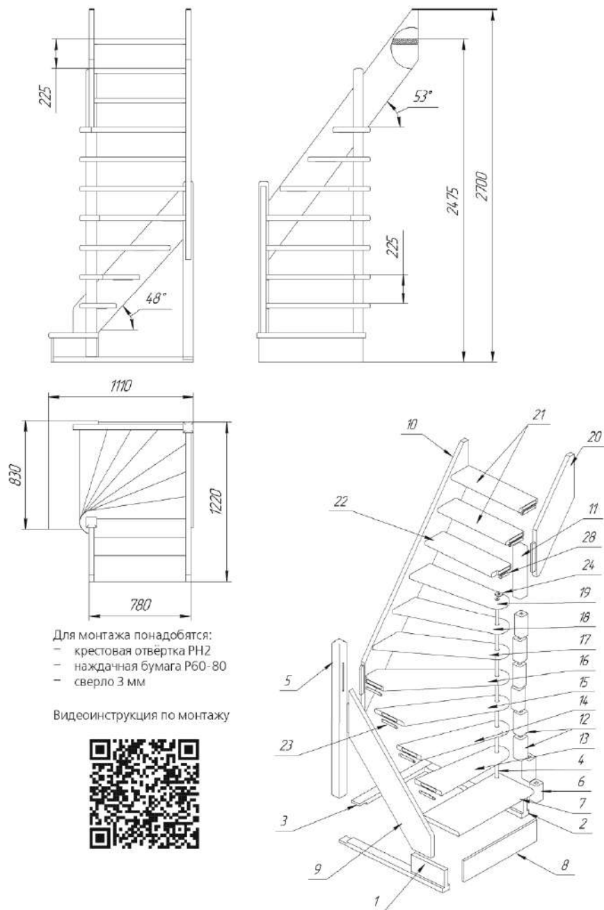
Рисунок 1. Лестница внутриквартирная ЛЕС-92..
